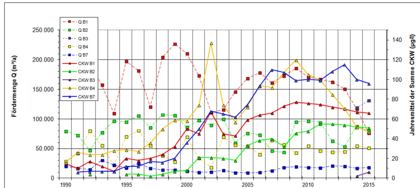
Bild 3 Entwicklung von CKW-Konzentration (µg/l) und Fördermenge (m³/a) in den Brunnen des WW Riedwiese
