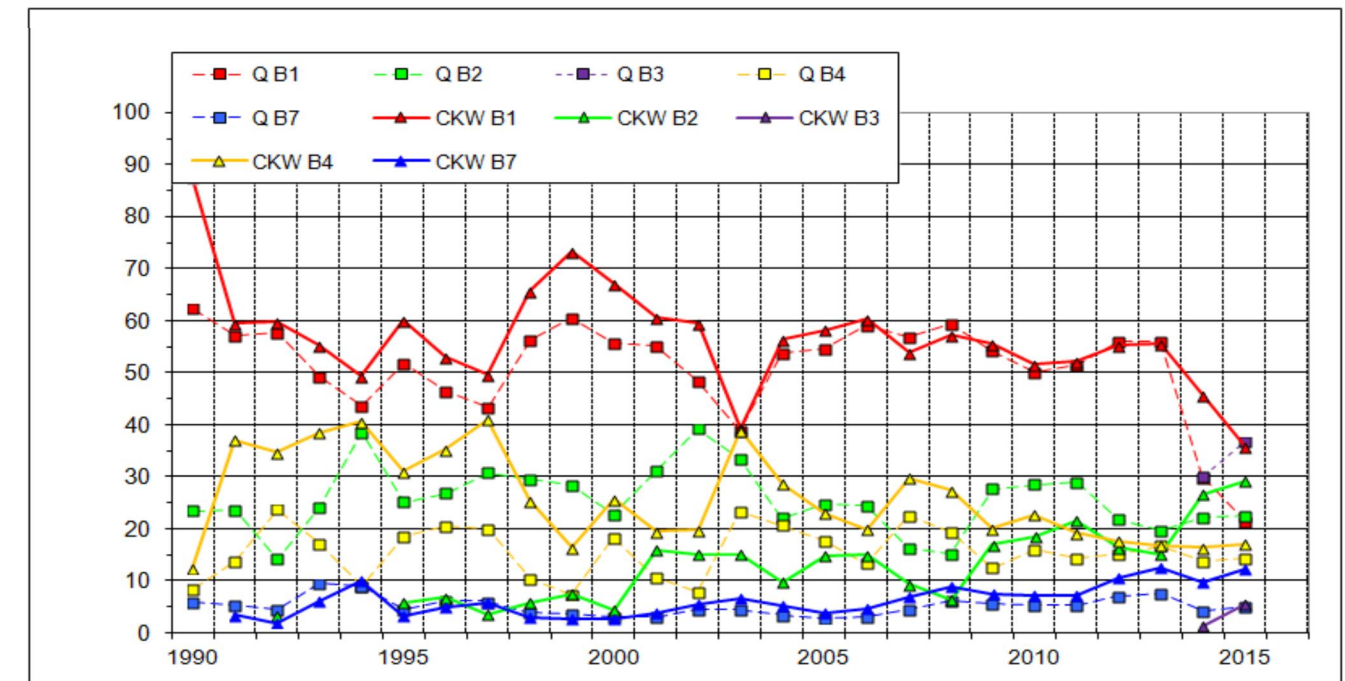
Bild 4 Entwicklung von CKW-Austrag und Fördermenge im WW Riedwiese (%)
