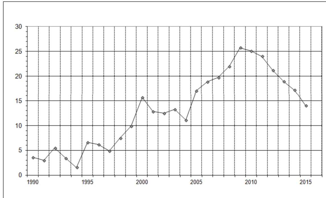
Bild 1 Entwicklung des CKW-Austrags im WW Riedwiese (kg/a), summarisch
