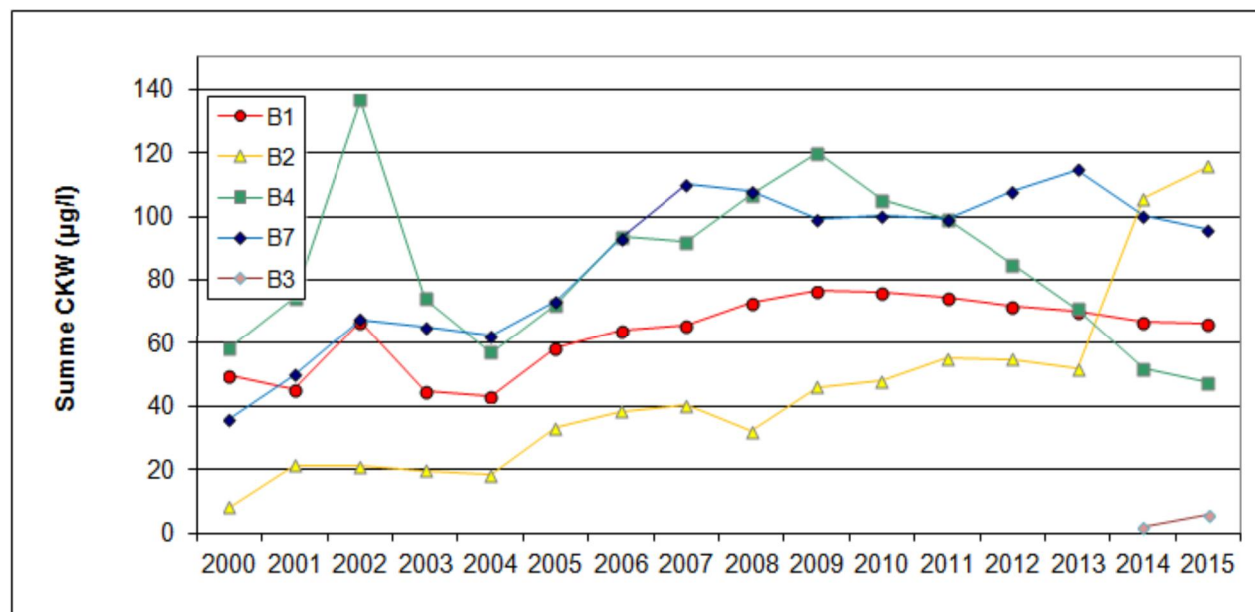
Bild 3 Arithmetische Jahresmittel der CKW-Kontamination WW Riedwiese
